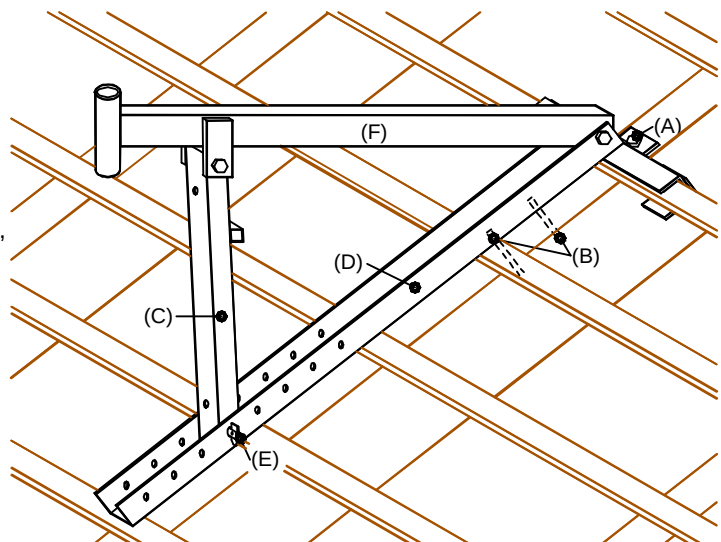
Bild 1 Grundaufbau
